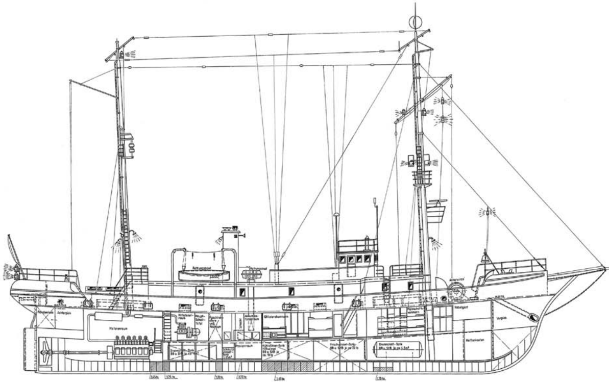
Schiffsriss von der ELBE 3
